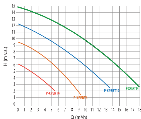
Výkonové křivky P-XPART
