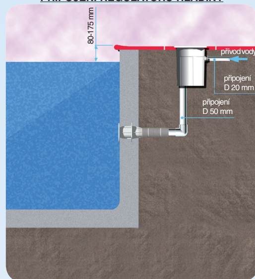
PŘIPOJENÍ REGULÁTORU HLADINY
