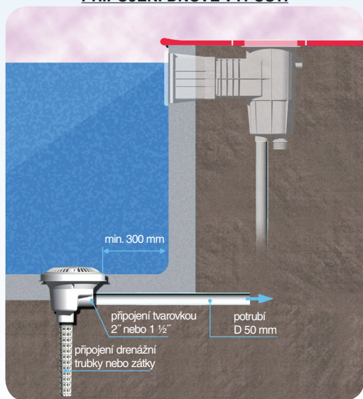
PŘIPOJENÍ DNOVÉ VÝPUSTI
