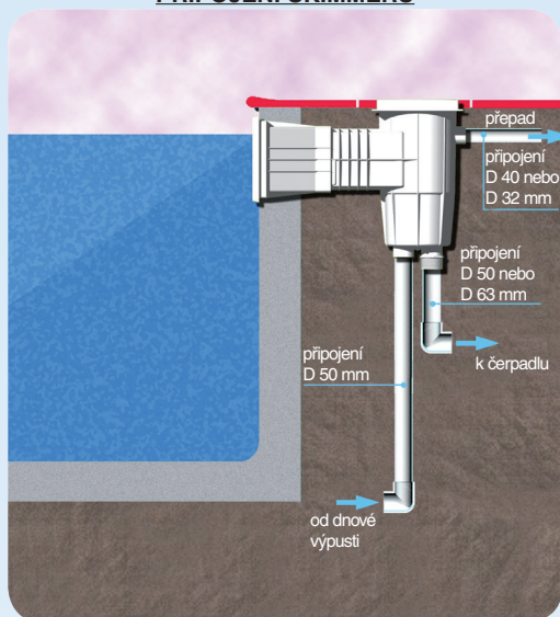
PŘIPOJENÍ SKIMMERU
