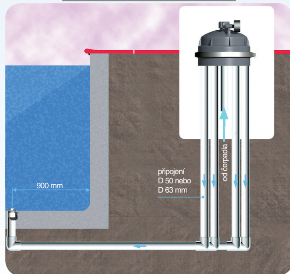
PŘIPOJENÍ TRYSKY NET'N'CLEAN
