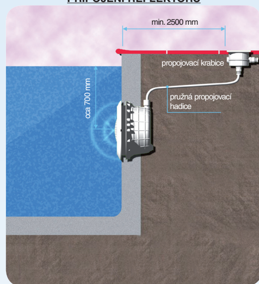
PŘIPOJENÍ REFLEKTORU
