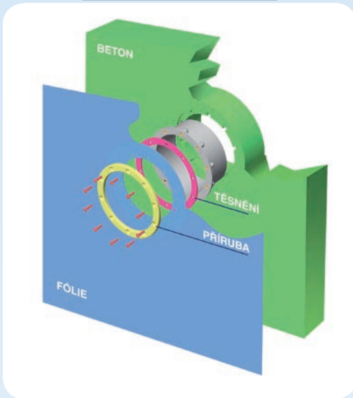
BETONOVÝ BAZÉN S FÓLIÍ
