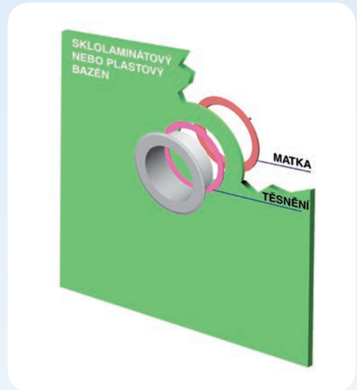
BAZÉN Z PLASTOVÝCH PANELŮ
