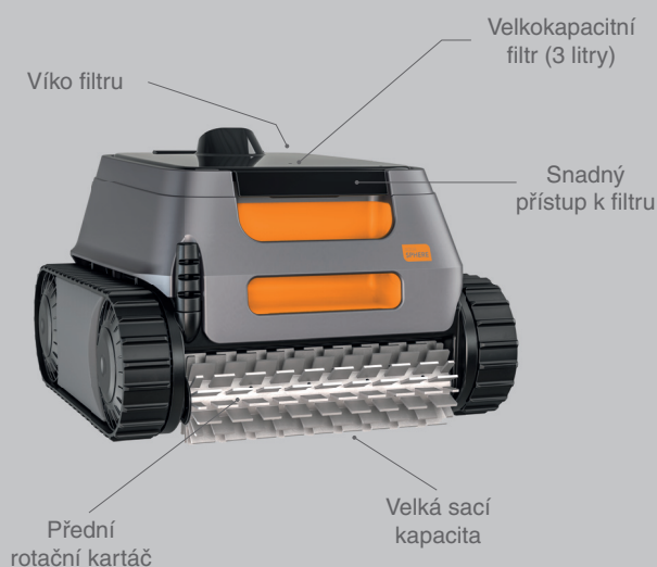
Cyklonové sání
