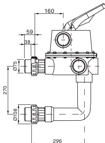
ovládací ventil Magnum 2½"
