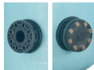
nová příruba sendvičového provedení
