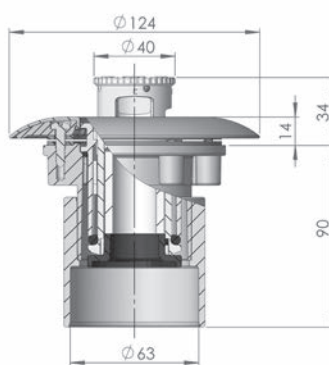
Tryska do fóliového bazénu
