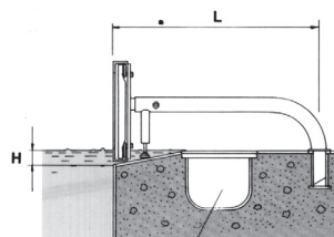
FINSKÝ TYP PŘELIVU
