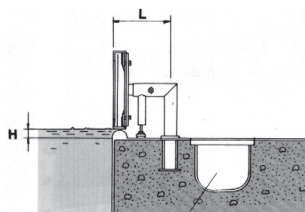
TYP ZURICH-WIESBADEN
