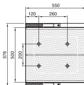
PŮDORYS (Kódy 28761 a 28760)
